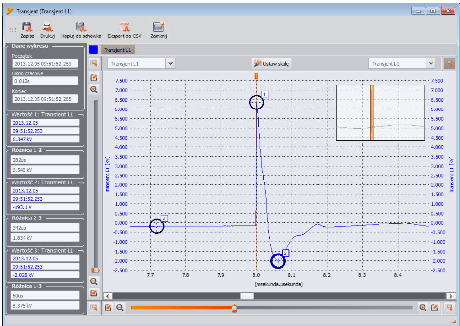
Rys. 54. Przykładowe przebiegi piorunowe.
