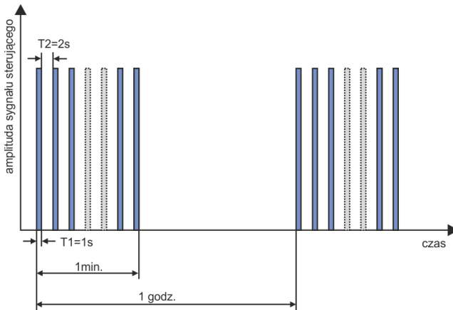
Rys. 48. Przykład transmisji sygnału sterującego niskiej częstotliwości.
